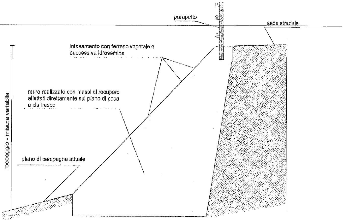
Roccaggio muro di sostegno
